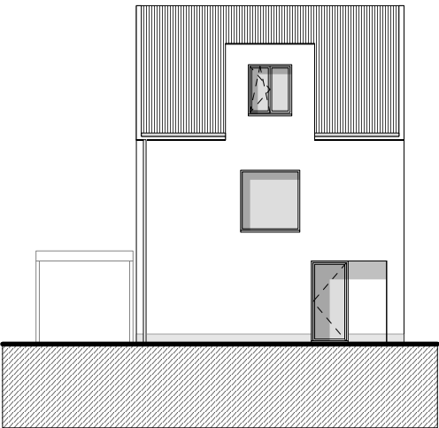
voorgevel
