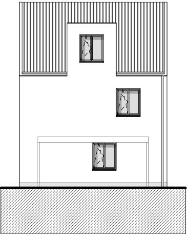
zijgevel links
