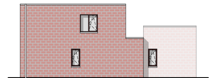
zijgevel rechts
