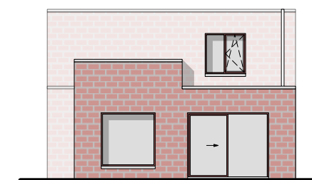
achtergevel
